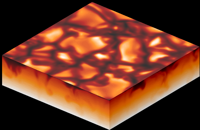
Sun
