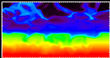
Sun
