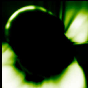
DUST
