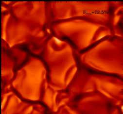
A-star
