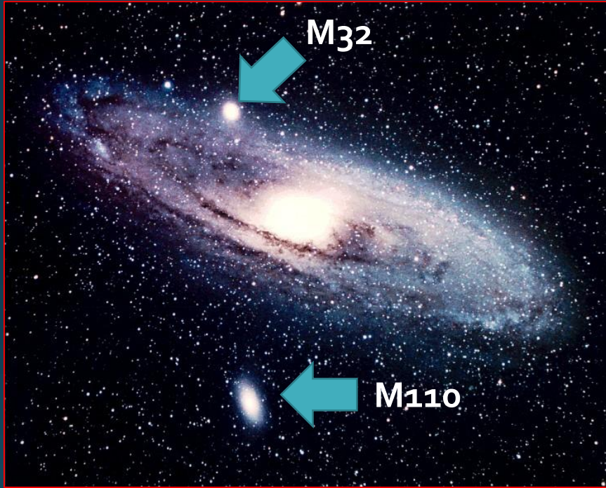
M31 (Andromeda)
