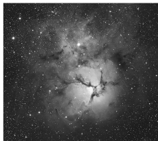
Trifidnebulosan uppvisar alla tre typerna av nebulosor; emission, reflektion och mörk.
