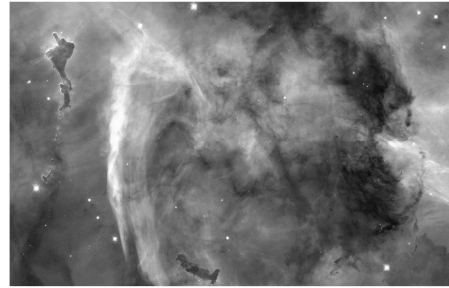
Carinanebulosan – ett typiskt stjärnbildningsområde (avstånd ca 8000 ljusår)
