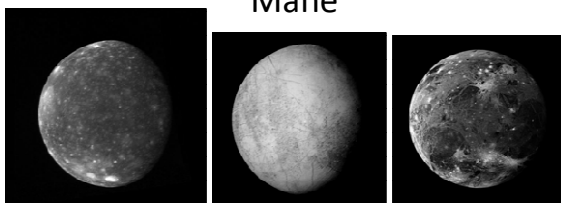
Callisto
