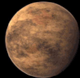
#5 Gliese 581 d
