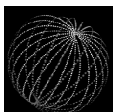
Dyson-svarm
