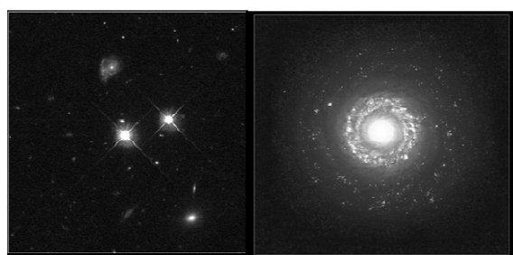
Kvasarer
