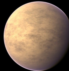
HD 40307 g*
