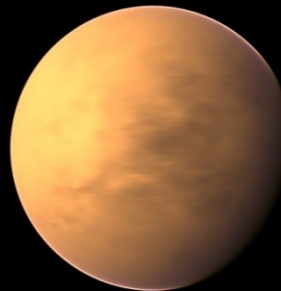
Gliese 163 c
