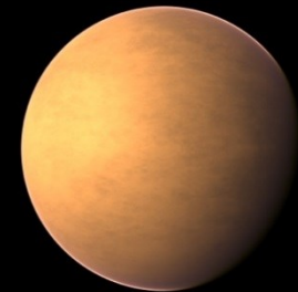
Gliese 581 d
