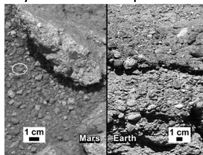
Curiositets fotografi av rundade stenar (t.v.), som verkar ha slipats i strömmande vatten
