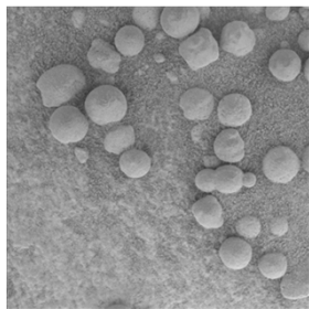
Hematit – tyder på förekomsten av flytande vatten i det förflutna
