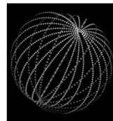
Dyson-svarm
