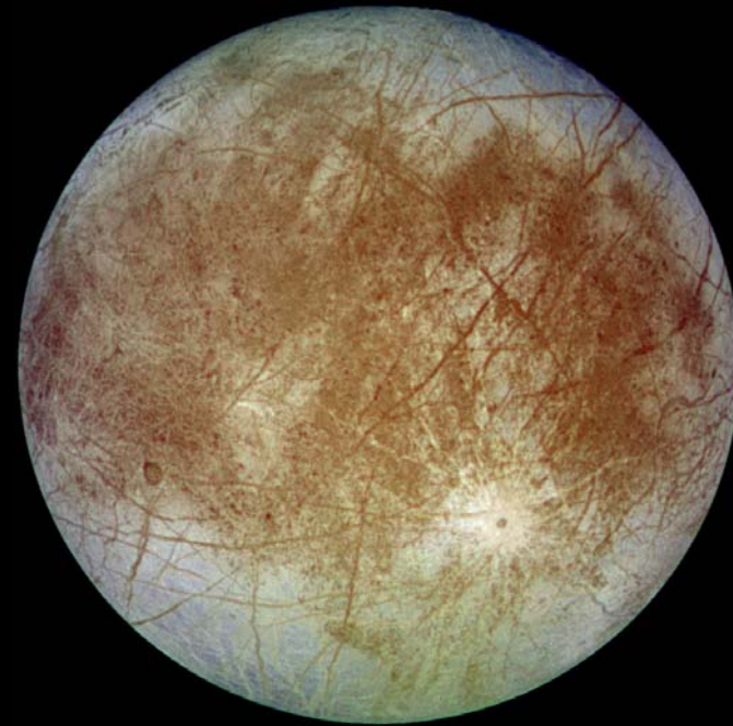
Jupitermånen Europa
