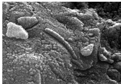
Fossila mikroorganismer från Mars i meteoriten ALH84001 som hittades i Antarktis 1984? Fortfarande oklart...
