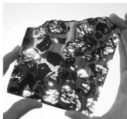
Delar av Fukang-meteoriten
