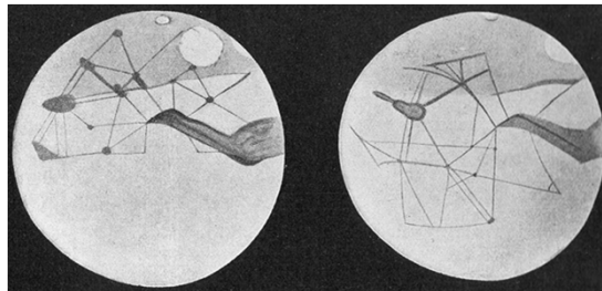
Percival Lowells kanaler, omkring 1890—1910
