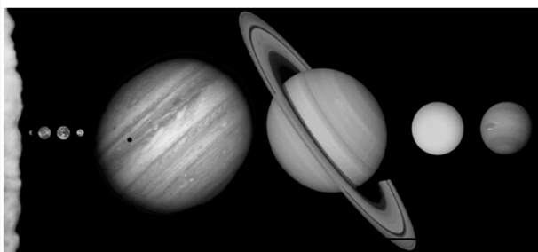
De inre (jordlika) planeterna
