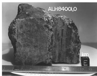
Marsmeteorit: Meteorit som slagits lös från Mars yta vid nedslag av asteroid eller komet, färdats genom rymden och slutligen fallit ned på jorden
