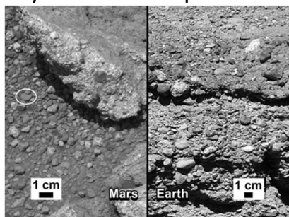
Curiositys fotografi av rundade stenar (t.v.), som verkar ha slipats i strömmande vatten
