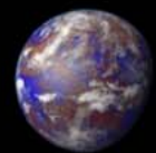
[12 ly] tau Cet e*
