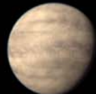
[16 ly] GJ 832 c
