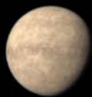
[13 ly] Kapteyn b
