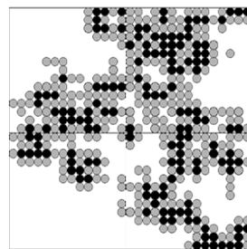
Perkolationsmodell
