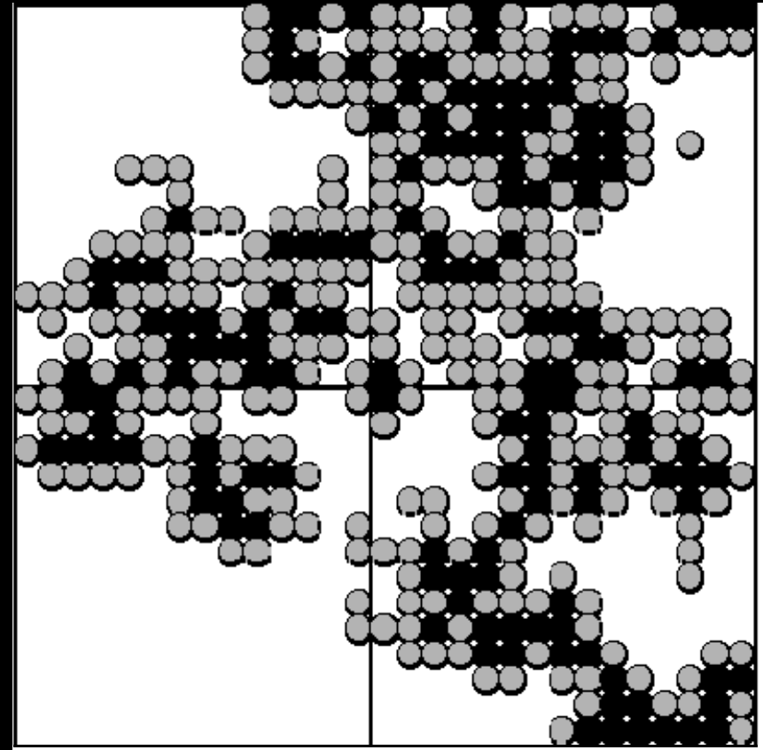
Perkolationssimulering
