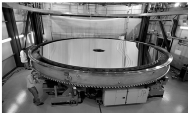
Spegeln (8.2 m) på Very Large Telescope (VLT)
