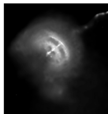
Pulsaren i Vela
