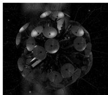
Konstnärlig vision av Bracewell-sond
