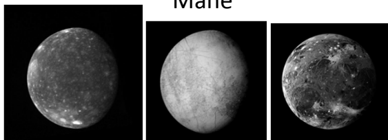
Callisto
