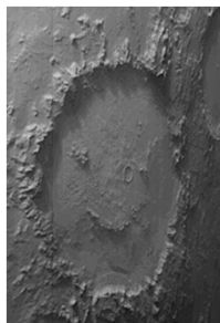
Galle-kratern
