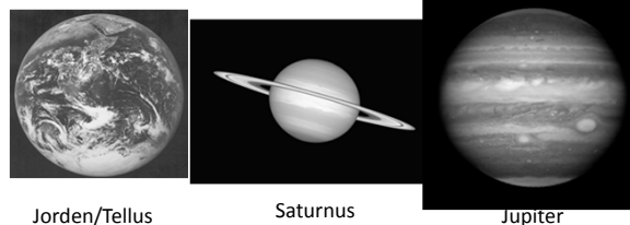
Jorden/Tellus
