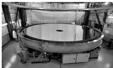
Spegeln (8.2 m) på Very Large Telescope (VLT)
